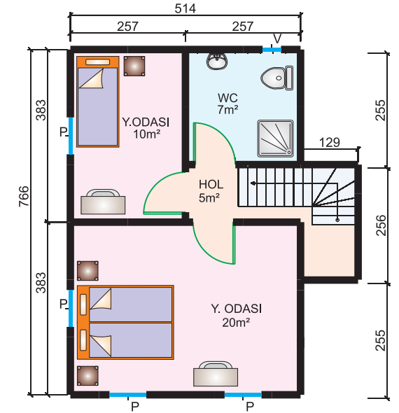
42 m 2 Üst Kat Planı
