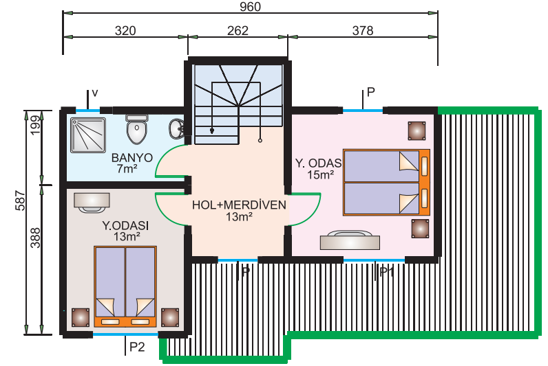
48 m 2 Üst Kat Planı
