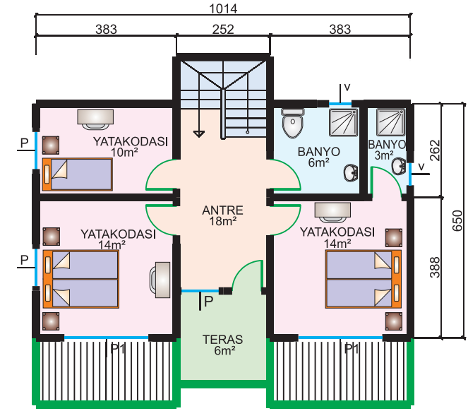
65 m 2 + 6 m 2 = 71 m 2 Üst Kat Planı
