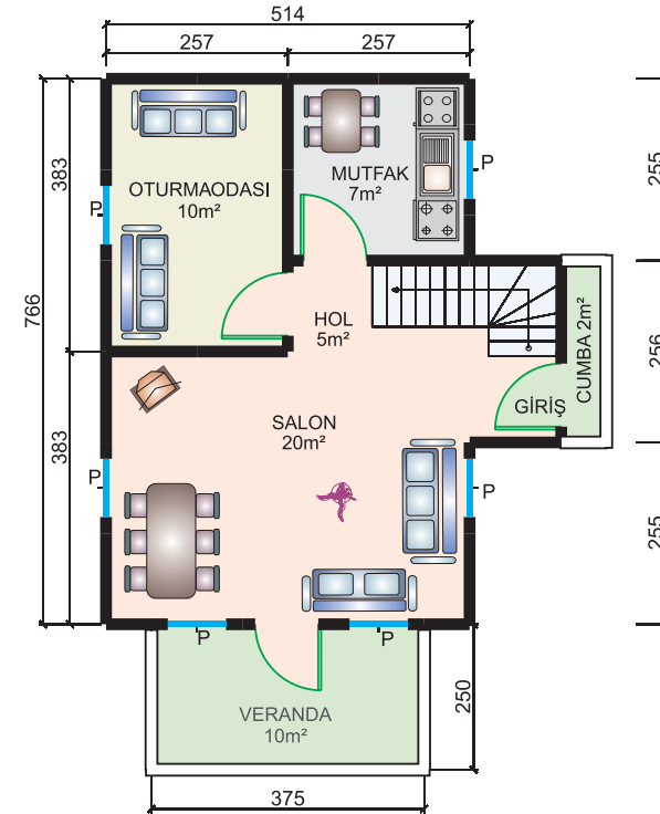
42 m 2 + 12 m 2 = 54 m 2 Alt Kat Planı
