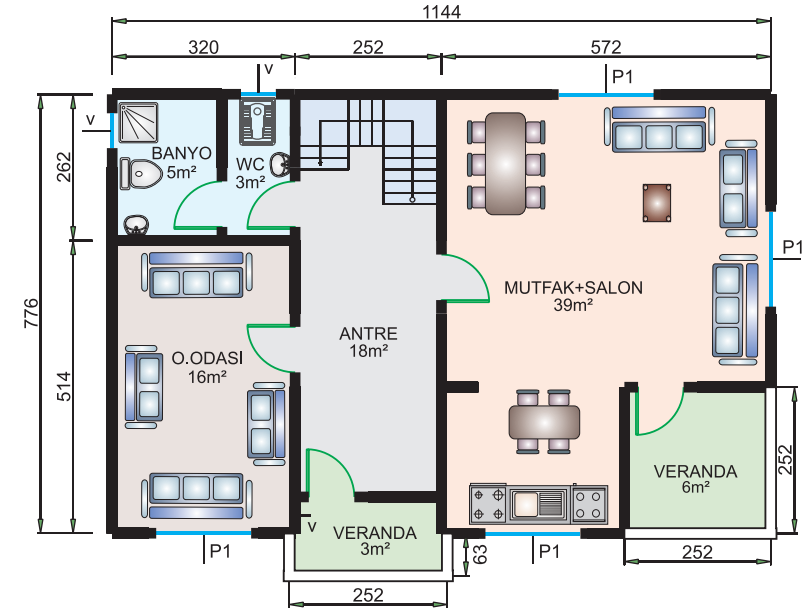
81 m 2 + 9 m 2 = 90 m 2 Alt Kat Planı
