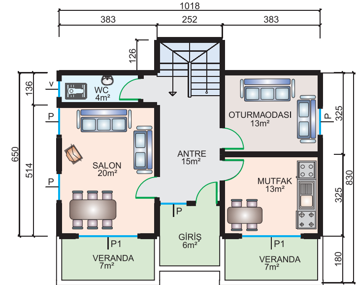
65 m 2 + 20 m 2 = 85 m 2 Alt Kat Planı
