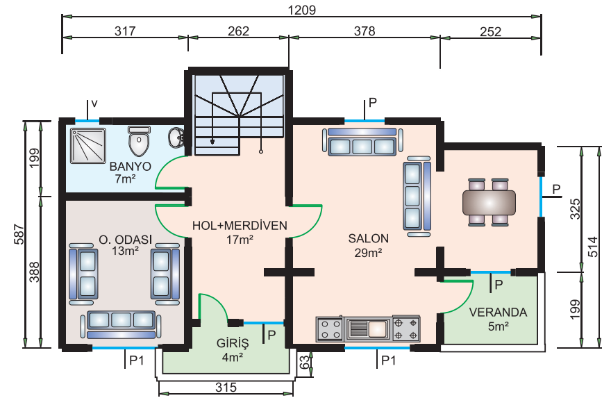
66 m 2 + 9 m 2 = 75 m 2 Alt Kat Planı
